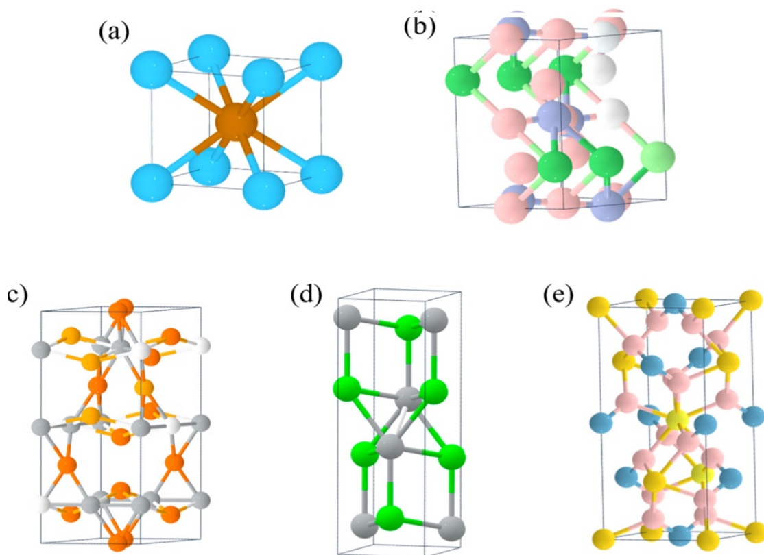
Figure 10.2: Crystal structure of (a) \text{FeTi} (b) \text{ZrNi} (c) \text{Mg}_2\text{Ni} (d) \text{NaAlH}_4 (e) \text{LiNH}_2
