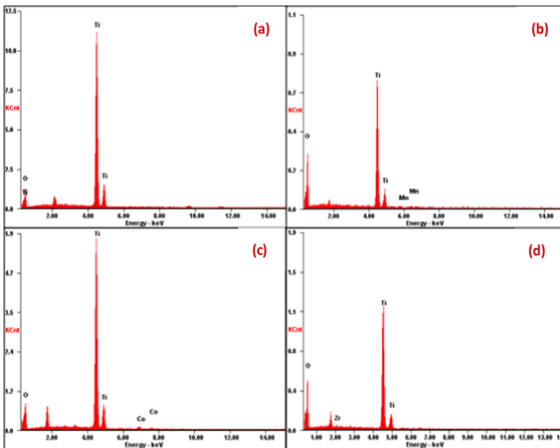
Fig. 5. EDS of a) pure TiO 2 , b) Mn doped TiO 2 , c) Co doped TiO 2 and d) Zr doped TiO 2 .
