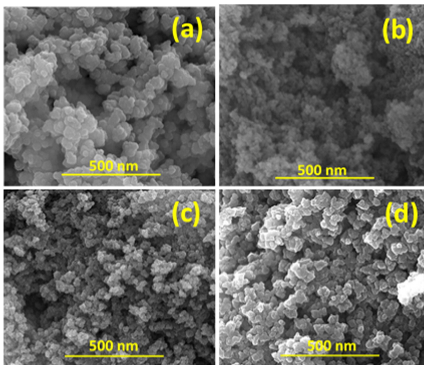
Fig. 4. FE-SEM images of a) pure TiO 2 , b) Mn doped TiO 2 , c) Co doped TiO 2 and d) Zr doped TiO 2 .
